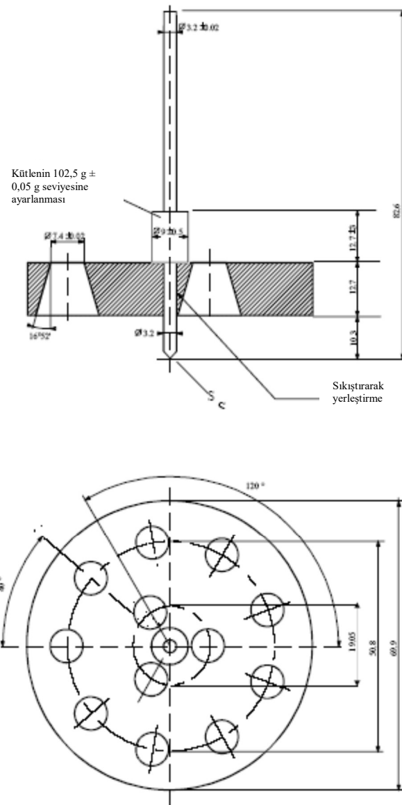
Şekil 1 - Penetrometre
